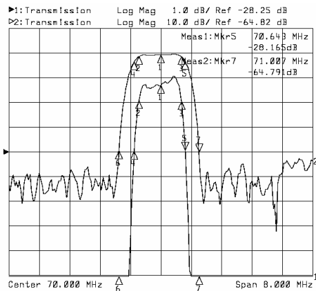
Horizontal: 0.8MHz/Div Vertical: 1&10dB/Div
